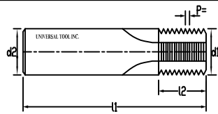
BSW
