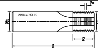
UNC
